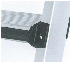
Geschraubte Stufen-Holm-Verbindung
